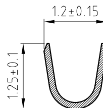
剖面 A-A
