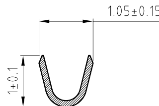
剖面 B-B
